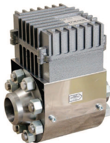
Рис. 16. Расходомер УРЖ2 КМ модель 3 ППД на высокое давление для пластовых вод
