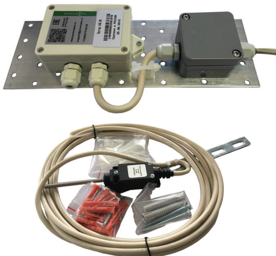
Рис. 14. Комплект «Датчик вскрытия люка и уровня-протечки PROMODEM GSM 830.04» для оперативного оповещения о возникновении аварийных ситуаций
