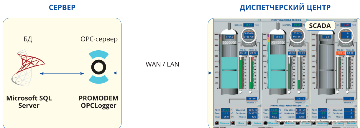
Рис. 18. Доступ SCADA-пользователя к архивам измерений и аварийных сообщений
